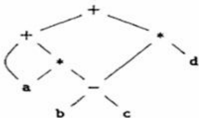
(a) DAG
