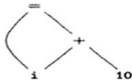
(a) DAG
